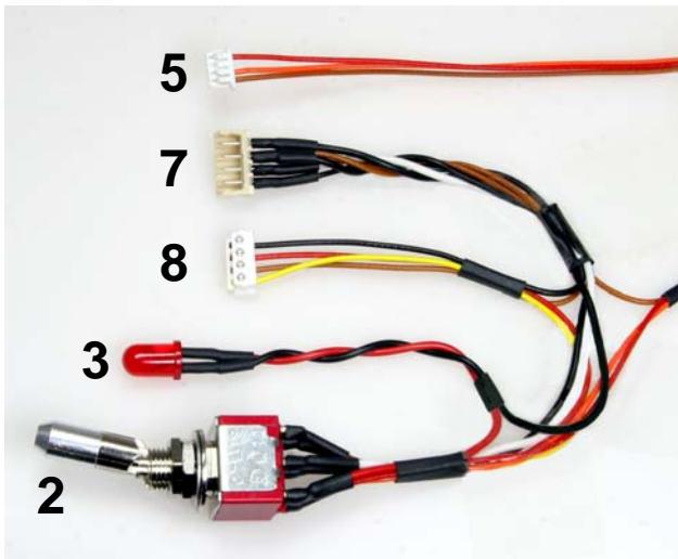
Original-Verdrahtung des alten Sendemoduls: Buchse (6) auf Stecker (9)
