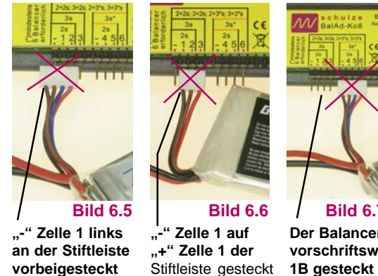
Bild 6.5, 6.6 und 6.7: Falsch-Anschlüsse
